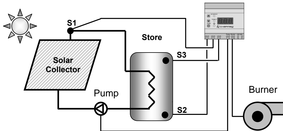
Σχήμα 1 Συνοπτικό σχέδιο εγκατάστασης Figure 1 Wiring Diagram
